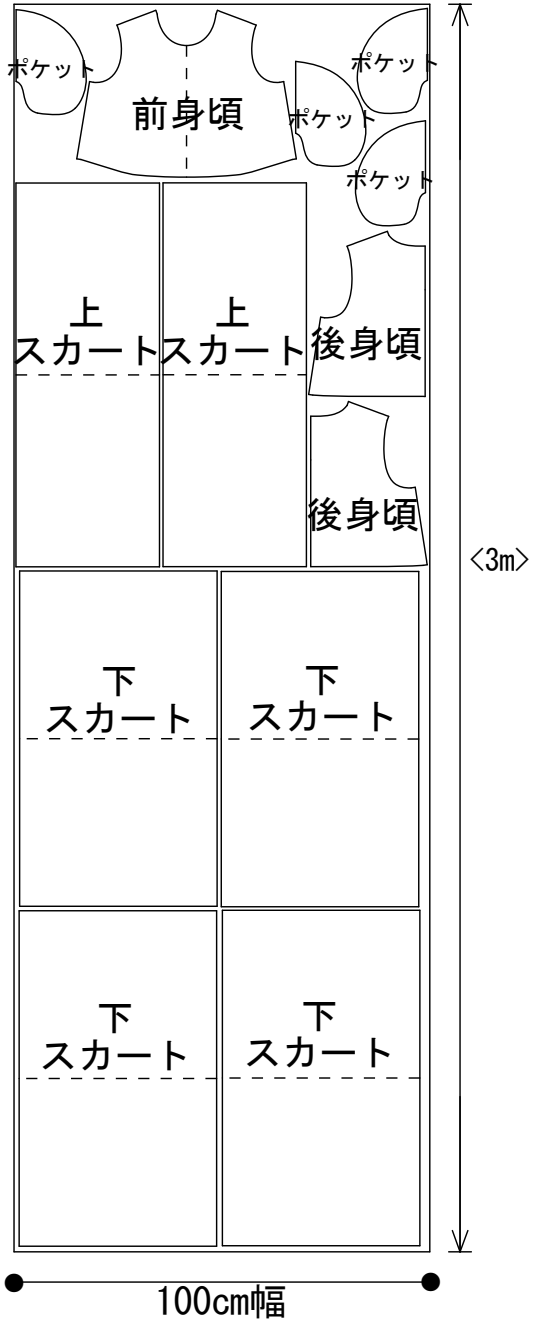
【36】 参考用尺 3m
