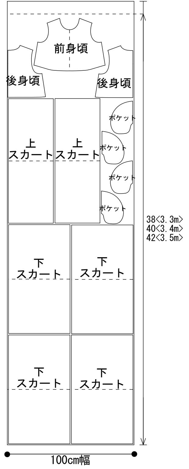
【38・40・42】 参考用尺 3.5m
