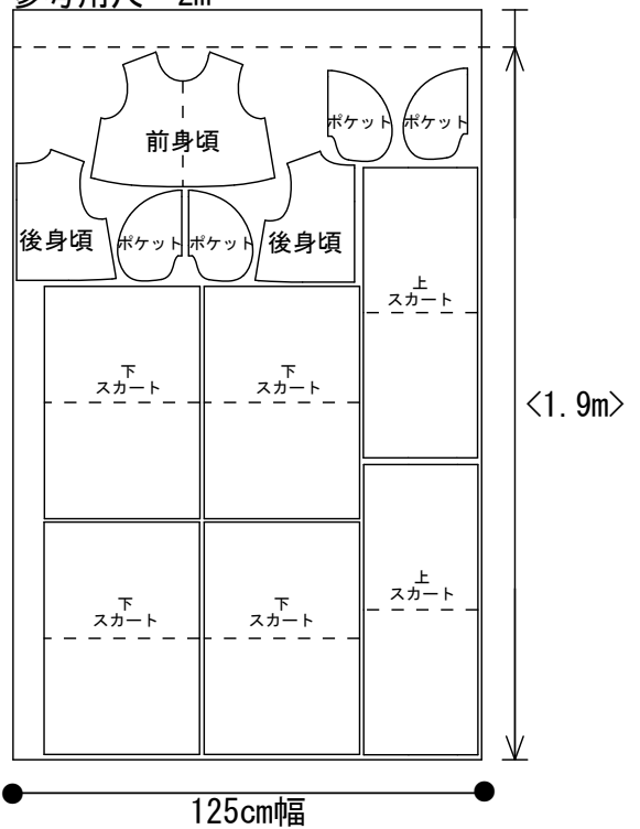
【14】 参考用尺 2m
